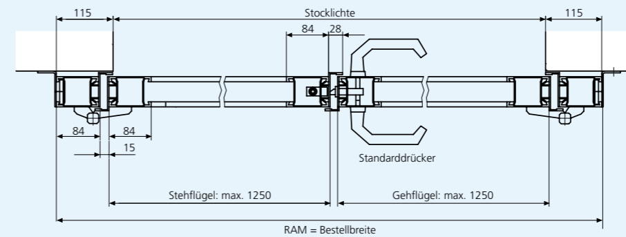
MONTAGE VOR ODER HINTER DER LAIBUNG
