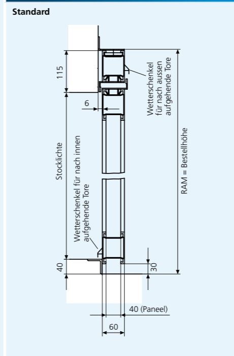
MONTAGE VOR ODER HINTER DER LAIBUNG
