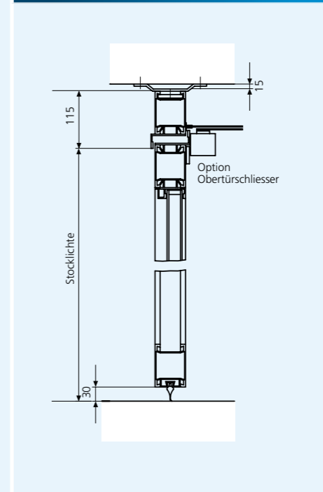
MONTAGE IN DER LAIBUNG
