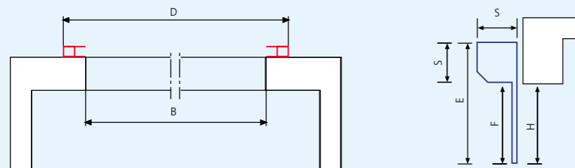
EINBAU LINKSROLLER AUSSEN AUF DAS MAUERWERK MONTIERT
