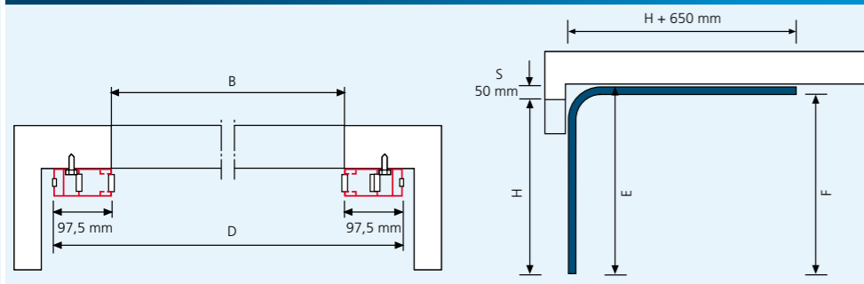
EINBAU HINTER DEM ANSCHLAG MONTIERT
