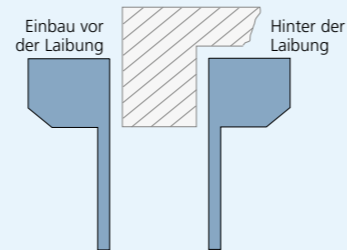
MONTAGEMÖGLICHKEITEN
