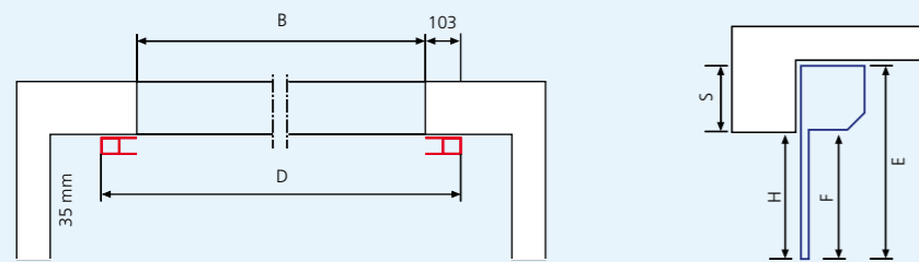
EINBAU RECHTSROLLER HINTER DEM ANSCHLAG MONTIERT
